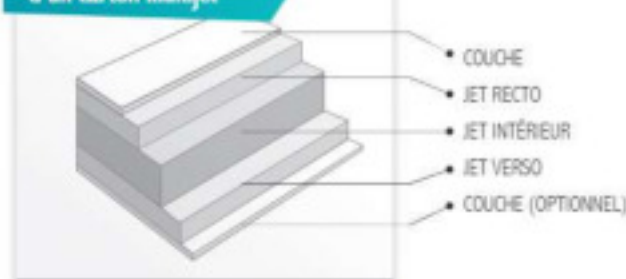
Coupe transversale d'un carton multijet
